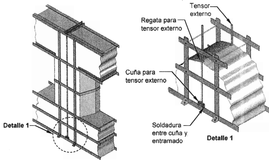
Figura 7.2.1.3-1 Tendores verticales externos sin anclaje a la cimentación.
