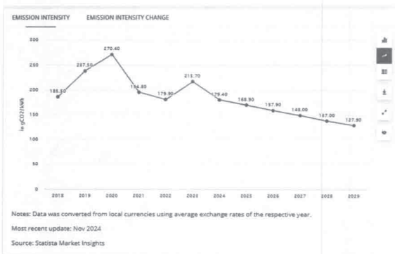
Gráfico 5 Intensidad de las emisiones en el sector energético en Colombia
